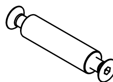
F[1SET] 8220-148 Ø20X74L
