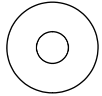
(C2)M8(I.D.)FLAT WASHER Ø24 QTY.6
