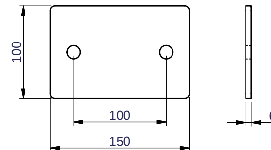
D [1PCS] 8313-027
