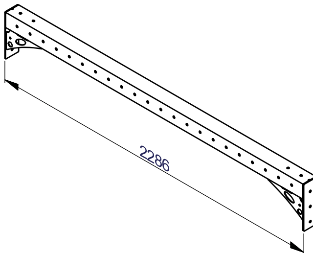
B1 [2SET] 20FMK2-A1
