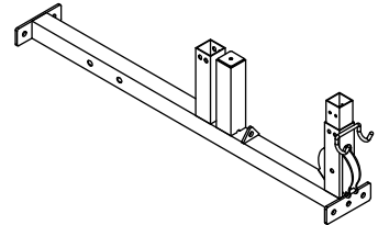
I[1PCS]
