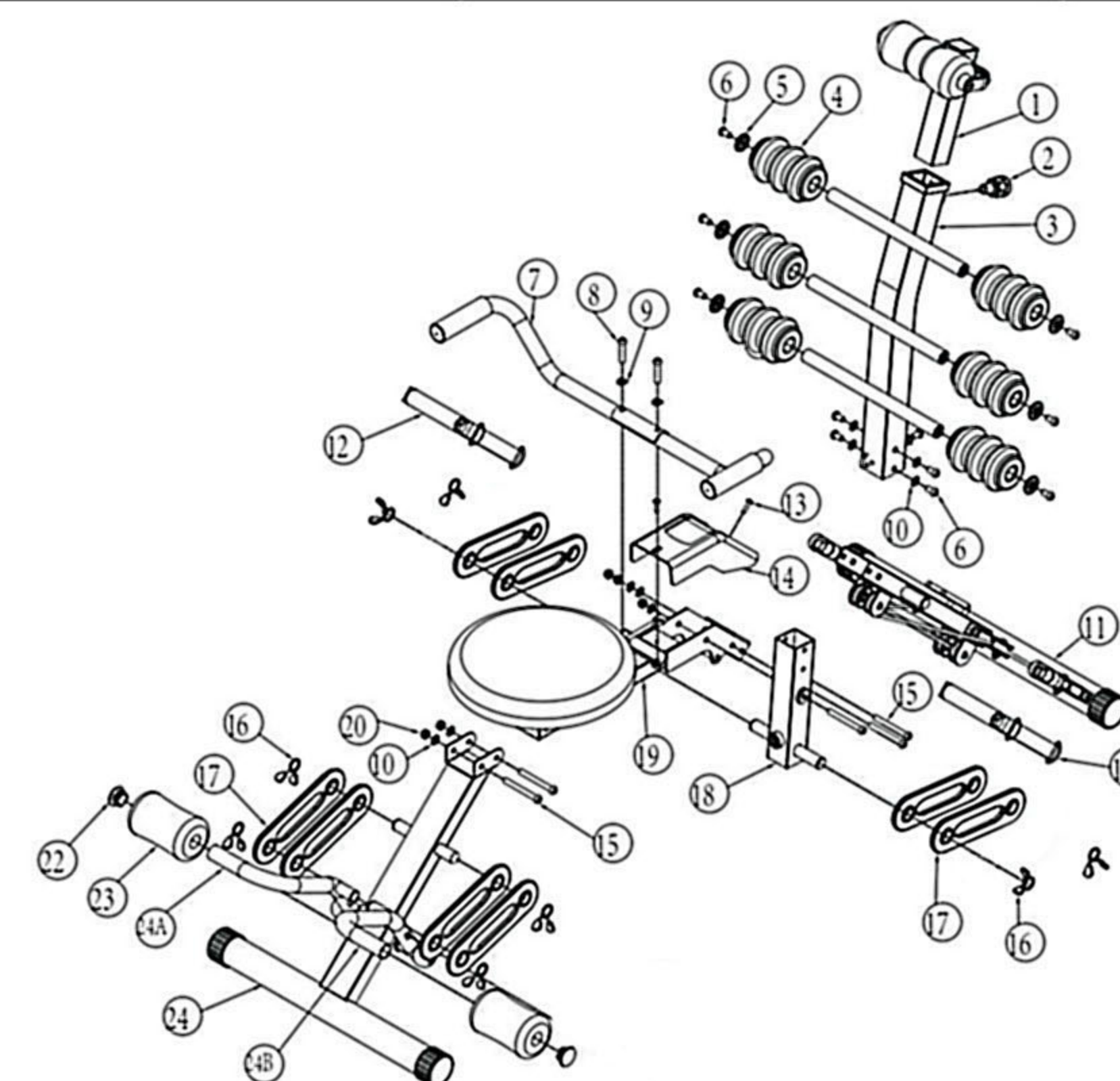
20.M8防松螺母 2PCS
